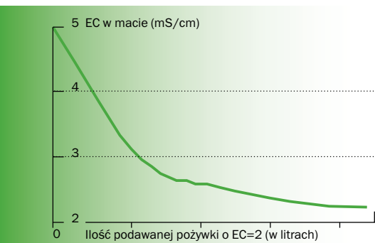
Pełna kontrola EC w macie (wyniki testów technicznych z laboratorium Grodan B.V.)
